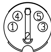
DIN 5-polig
