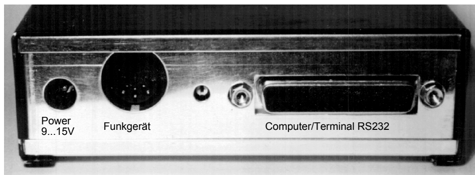
TNC21S, Rückseite
