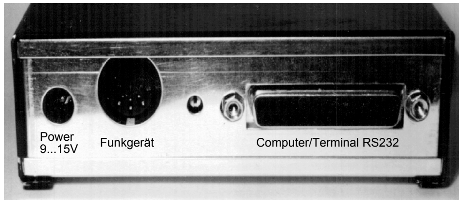
TNC21S, Rückseite
